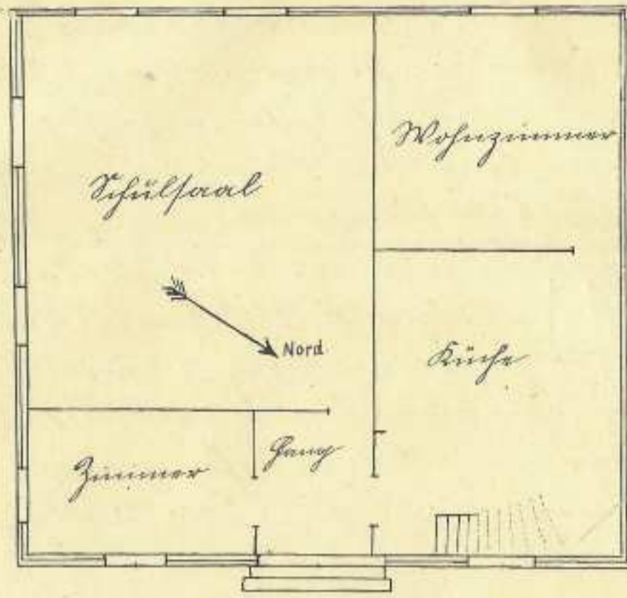
Grundriß des alten Tischstübchen (1:100).
