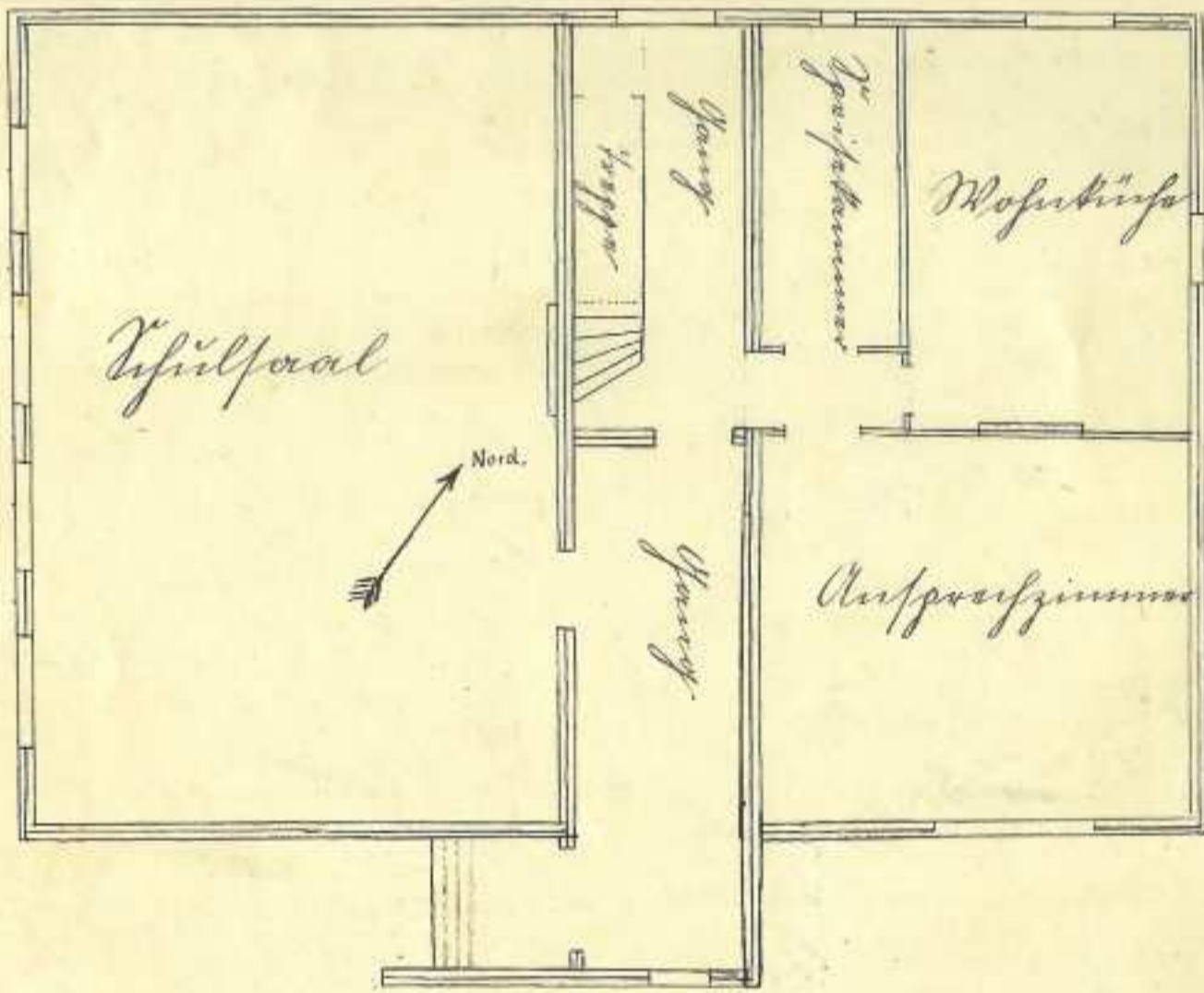
Grundriß des neuen Tischstübchen (1:100).
